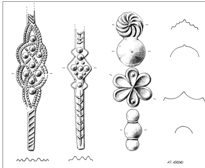
Fig. 2. De gjutna produkterna i plan och profil. Skala 1/1. Ritning: Anders Eide, Stockholm.
